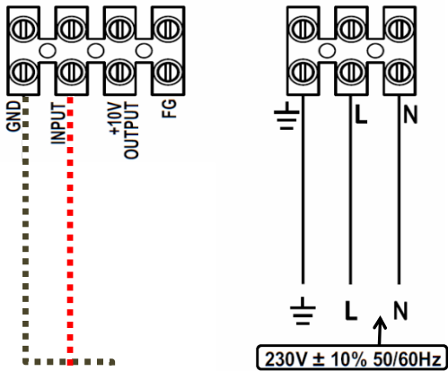
Aansluitschema buisventilator:
