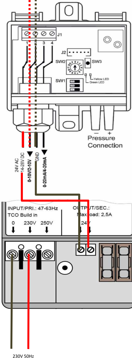
Aansluitschema pressostaat TDP-D:
