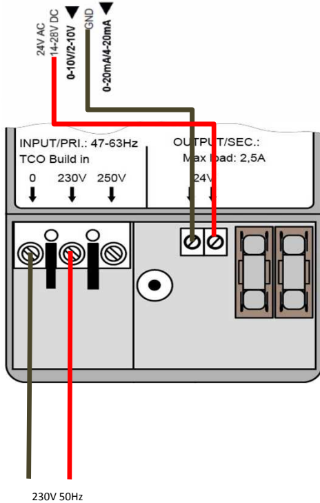
Aansluitschema TRAF060:
