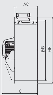
Korte behuizing (C en CK) - tot IEC 200 Alleen met aansluitdoos (CK) - vanaf IEC 225
