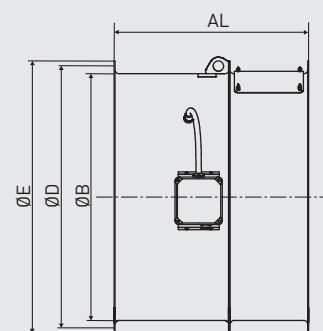
Lange behuizing (LPK) THGT 900 tot 1250
