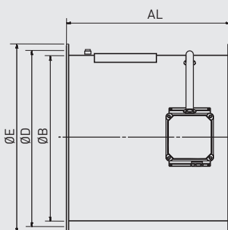
Lange behuizing (LK en LPK) THGT 400 tot 800
