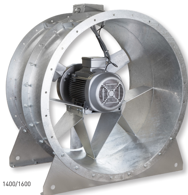
Lang Frame (behuizing) (L-versie)
