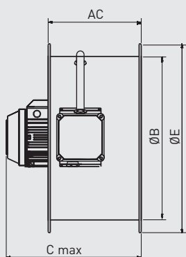
Korte behuizing (CK) THGT 400 tot 1250
