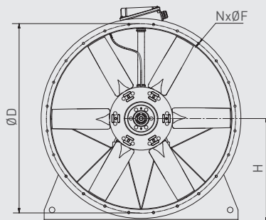
Lange behuizing (LP, LK en LPK) - tot IEC 200 Alleen met aansluitdoos (LK en LPK) - vanaf IEC 225
