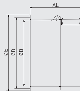
Lange behuizing (LP) THGT 900 tot 1250
