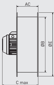
Korte behuizing (C) THGT 400 tot 1250
