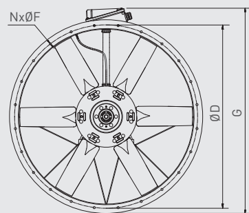
Korte behuizing (C en CK) - tot IEC 200 Alleen met aansluitdoos (CK) - vanaf IEC 225
