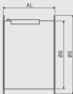
Lange behuizing (LP) THGT 400 tot 800
