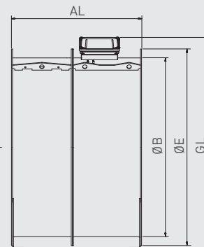
Lange behuizing (LP, LK en LPK) - tot IEC 200 Alleen met aansluitdoos (LK en LPK) - vanaf IEC 225
